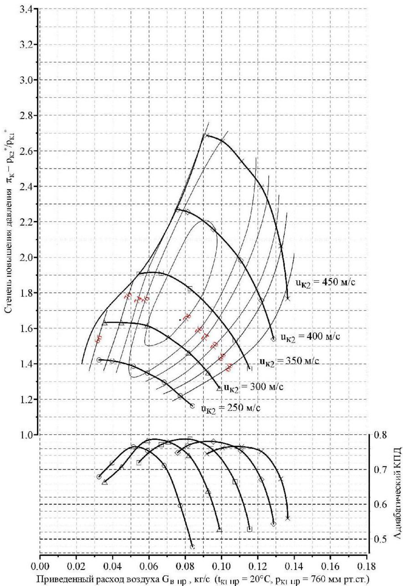
Характеристики компрессора ТКР 50.07.10
